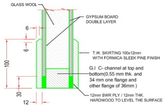
DETAIL D2
